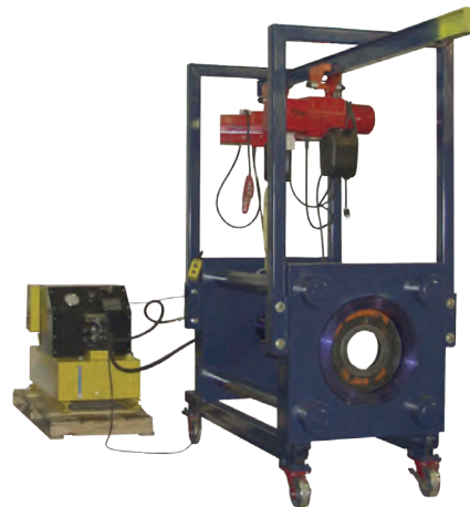
350 Ton Ram
